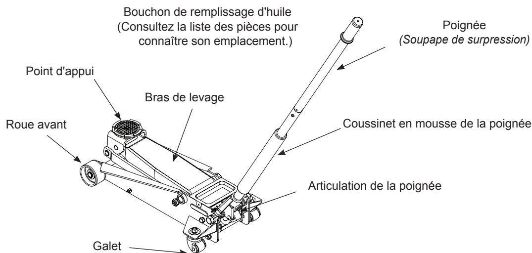
Figure 1 : Pièces d'un cric type
