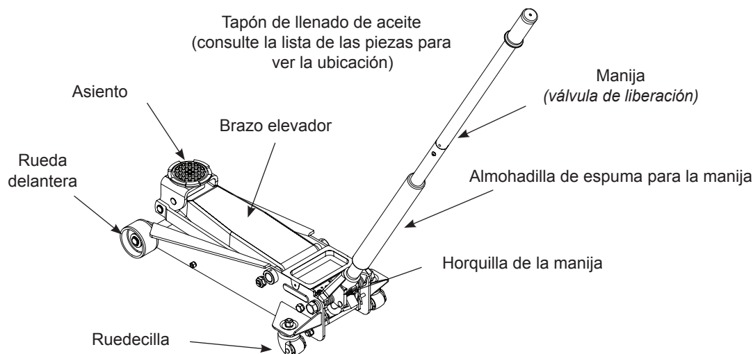
Figura 1: Nomenclatura habitual de un gato
