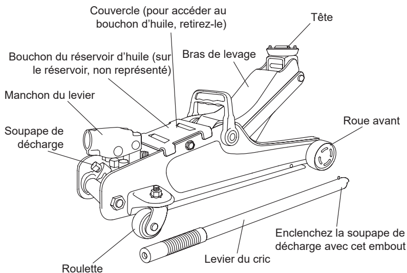
Figure 1 - Nomenclature typique du cric rouleur
