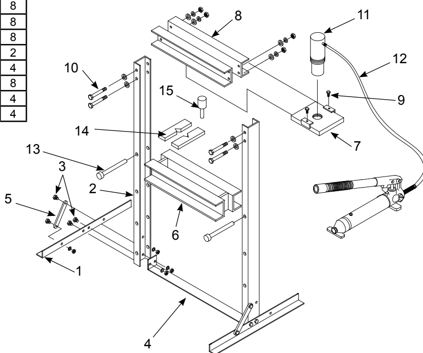
Figure 6 - Illustration d'assemblage du modèle 65123
